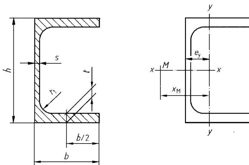
شکل ۱- مقطع عرضی ناودانی
